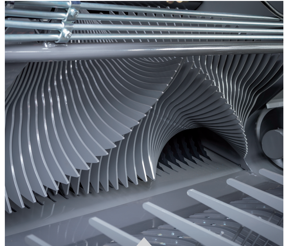
Schneidwerk mit 25 Messern
