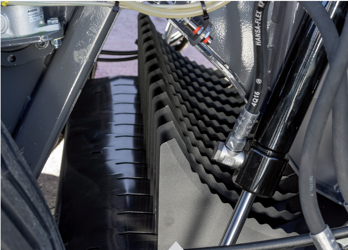
Die MF RB 3130F kann mit einem Xtracut -Schneidwerk mit 13, 17 oder 25 Messern ausgestattet werden.
